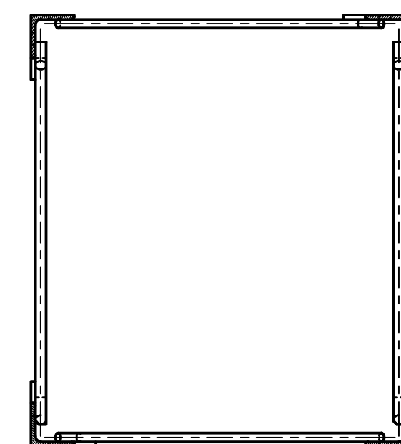
Typisk snitt C-C
